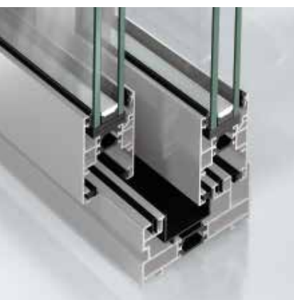
Раздвижная система Schüco ASS 48 Schüco sliding system ASS 48
