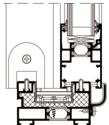
Раздвижная система Schüco ASS 43, масштаб 1:2 Schüco sliding system ASS 43, scale 1:2
